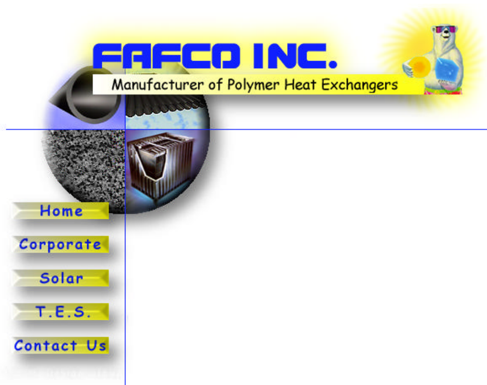
-web gui-
