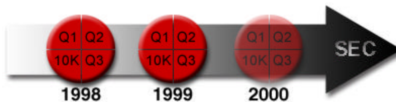
-web gui-
